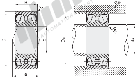
安装图
