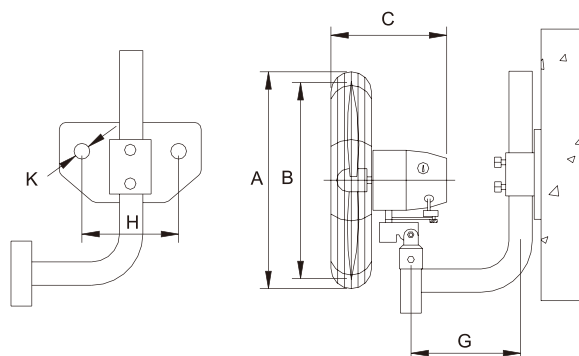
挂墙式外形尺寸图
