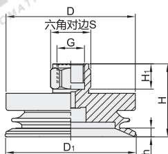
内接螺纹 外形B
