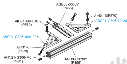
分解图
