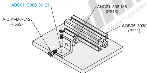
分解图
