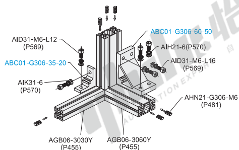
分解图
