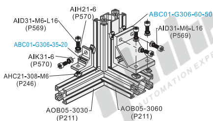
分解图
