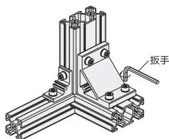
组装图
