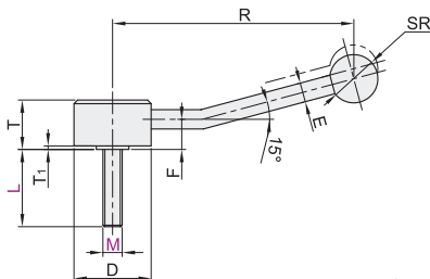
角形手柄型 HAG71
