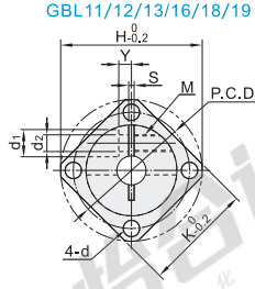
方法兰型 GBL11/12/13/16/18/19
