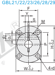
对边法兰型 GBL21/22/23/26/28/29
