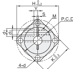
方法兰型 GBJ11/12/13/16/18/19
