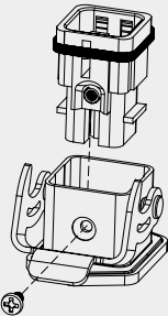
安装示意图
