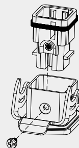
安装示意图
