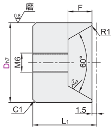
外安装型·加长型
