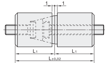
组装尺寸
