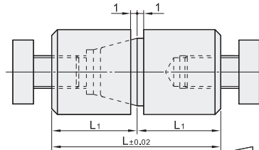
组装尺寸
