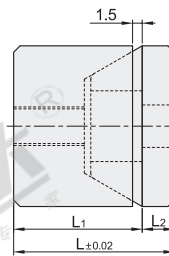
组装尺寸
