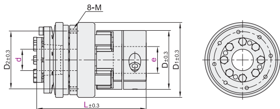
一端免键另一端螺钉夹紧 DEP82
