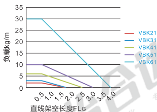
直线架空长度与负载关系图FLg
