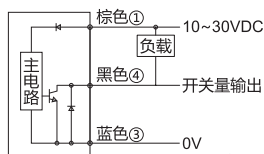
NPN输出
