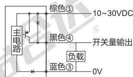
PNP输出
