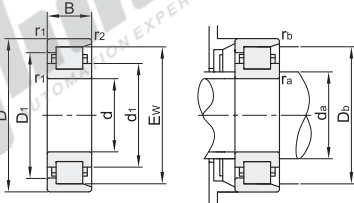
NF：外圈单挡边，内圈双挡边
