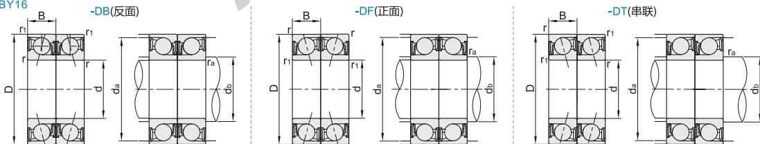
高速单列角接触球轴承
