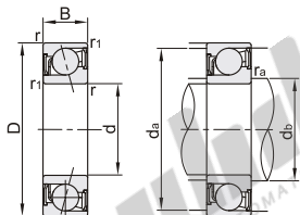
高速单列角接触球轴承 BBY06
