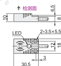
外壳尺寸: Q18C(18×10)
