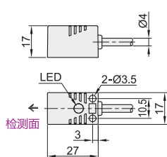
外壳尺寸: Q17(17×17)
