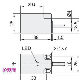
外壳尺寸: Q25(25×25)
