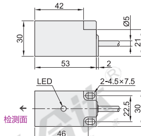
外壳尺寸: Q30(30×30)
