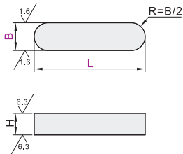
A型 Y-LBA02
