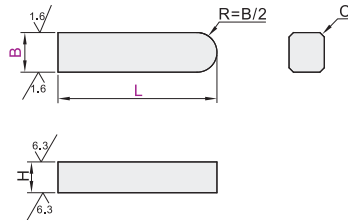
C型 Y-LBA06
