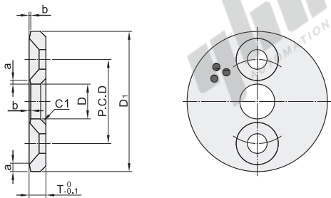
锥孔型(内六角沉头螺钉用) OFU01
