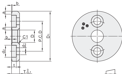
沉孔型(内六角薄圆柱头螺钉用) OFU02
