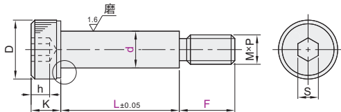
L尺寸指定型 PACK-TBH05/42
