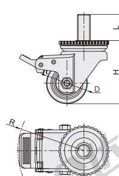
塑料单刹 CEL52
