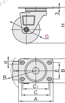
平底活动型 CFL01
