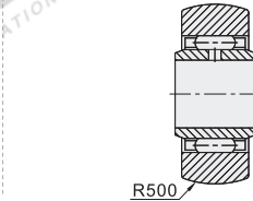
球面型 BPS25/26
