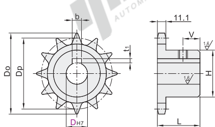
链轮 VLY31/32
