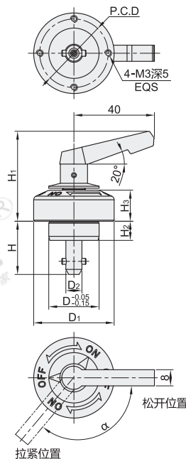
手柄型·圆柱销 HCD08
