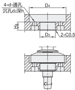
安装方式B
