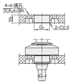
安装方式A
