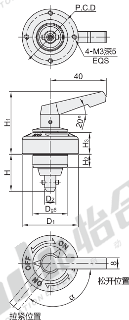
手柄型·圆锥销 HCD07
