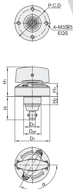
旋钮型·圆锥销 HCD05
