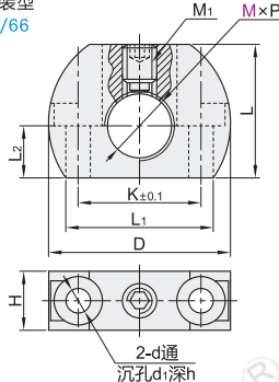
垂直安装型 ZAF65/66
