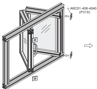
组装图
