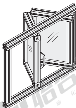
组装图
