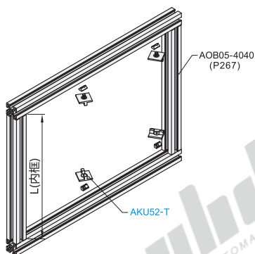
分解图
