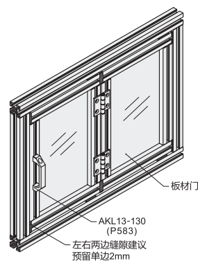
组装图
