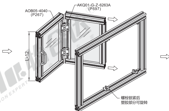
组装图
