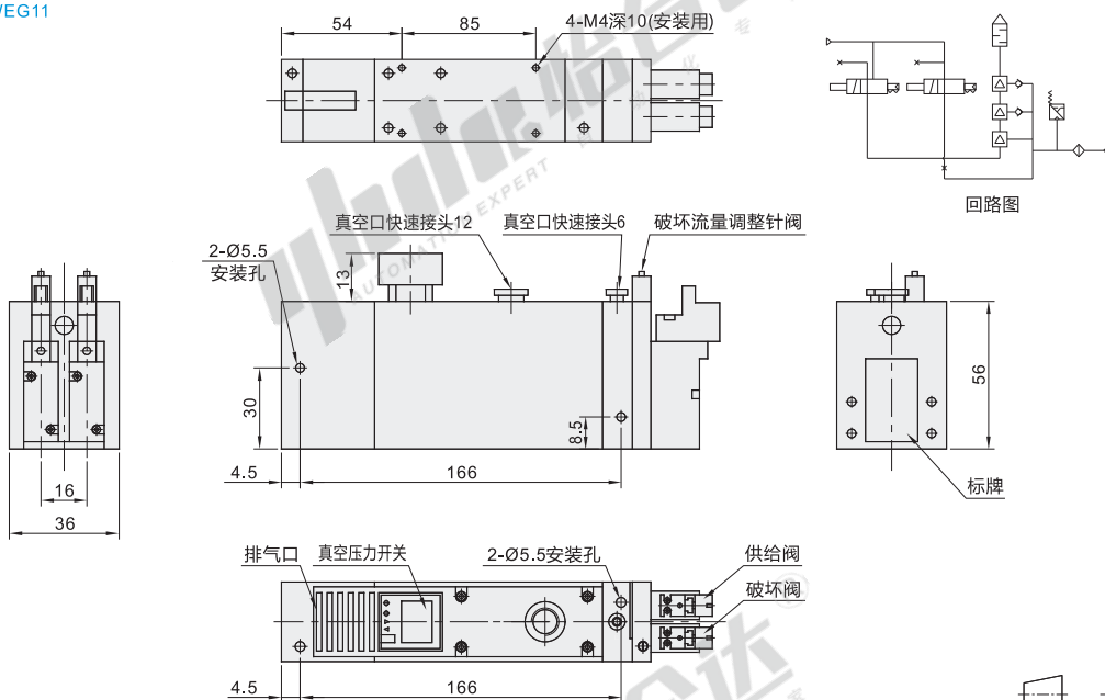
带真空压力开关、带阀组合 WEG11
