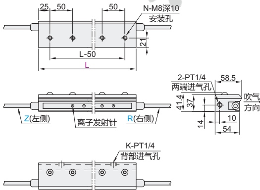
高速平行出气 ZWB71
