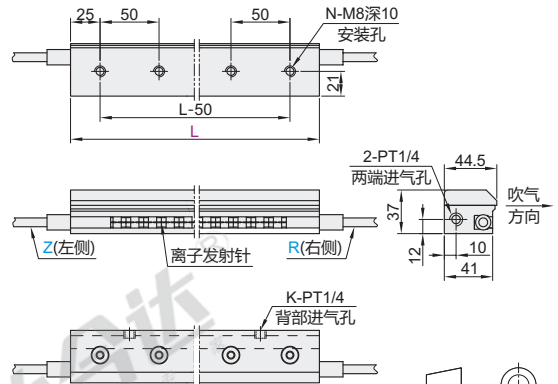
平行出气 ZWB72
