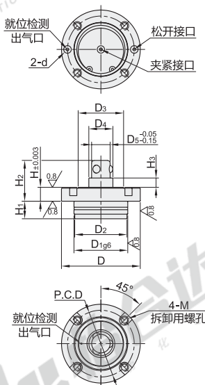
圆柱销 HCD22
