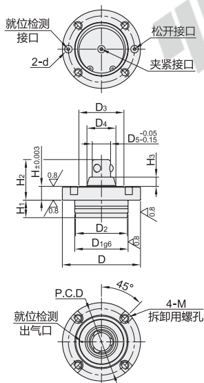
圆锥销 HCD21
