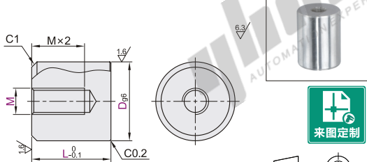
板材定位销
