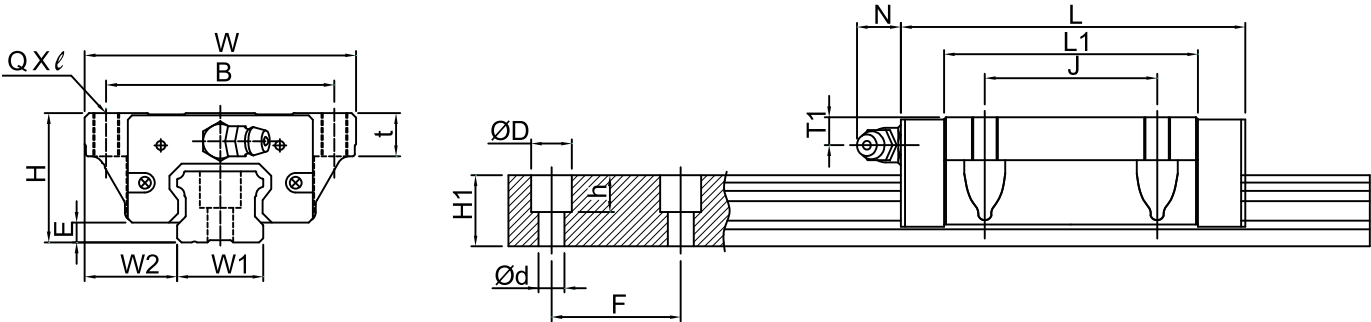
TRH-F 高組裝系列規格尺寸表
