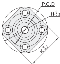
方法兰 BFP41/42/46/71/72
