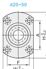
对边法兰 BFP51/52/53/54/56/81/82/83
