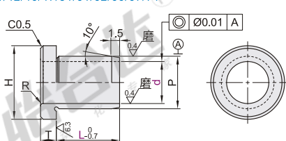
带肩型·薄壁型
