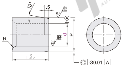
带肩型·标准型
