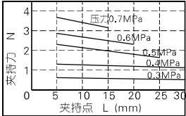
HFTZ10\HFTK10
