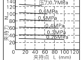
HFSZ32\HFSK32
