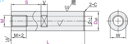
一端内螺纹带扳手槽型 E-SLD21
