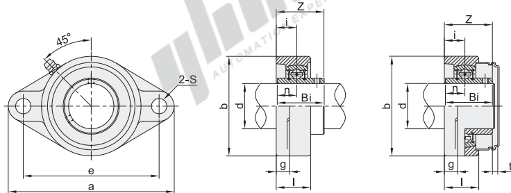
标准型 UCFL....-FKB
