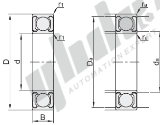
安装图
