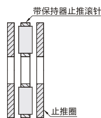
组件 带保持器止推滚针+止推圈 E-BBL
