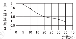
最大加速度VS负载
