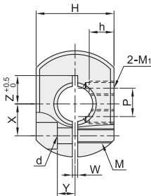
开口型-紧定螺钉锁紧型 FBA11/12/16
