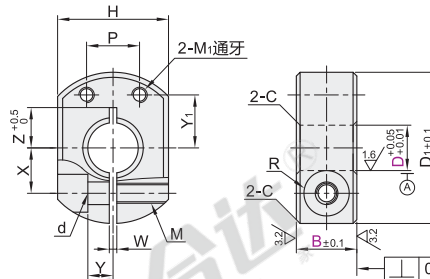
开口型-侧安装型 FBA21/22/26
