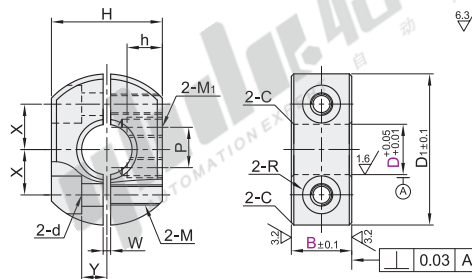
分离型-紧定螺钉锁紧型 FBA61/62/66
