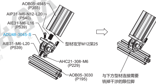
分解图
