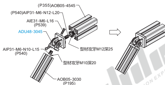
分解图
