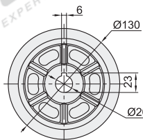
键槽孔型 CNG11
