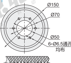
轮面斜纹分布平面图
