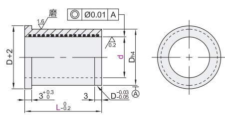
肩型(材质: FC250+MoS 2 ) OFC22
