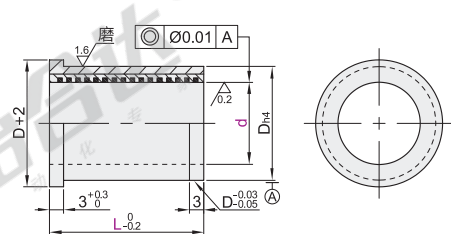
肩型(材质: SUJ2+铜合金+MoS 2 ) OFC32
