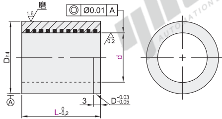
直柱型(材质: FC250+MoS 2 ) OFC21
