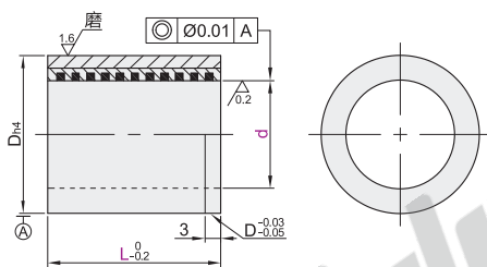
直柱型(材质: SUJ2+铜合金+MoS 2 ) OFC31
