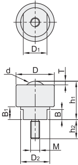
标准型(SCM415H) QDE61
