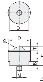
标准型(SUS304) QDE64
