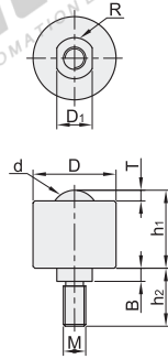
标准型(S45C) QDE60
