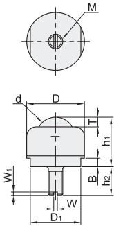
标准型(SCM415H) QDE61
