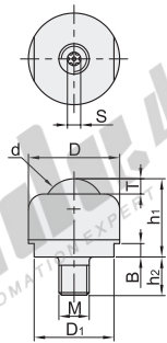
垃圾孔排出型 QDE62
