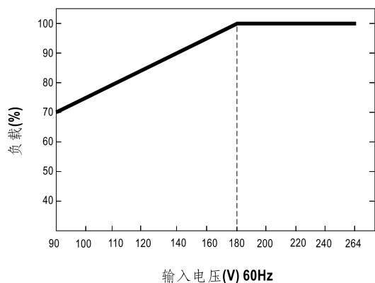
■ 降载曲线
