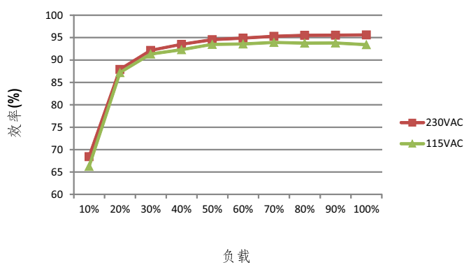
■ 效率VS负载(48V机型)
