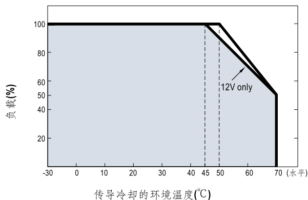
■ 降载曲线
