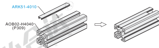
分解图
