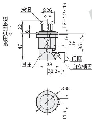
转动按钮型 XBF01/02
