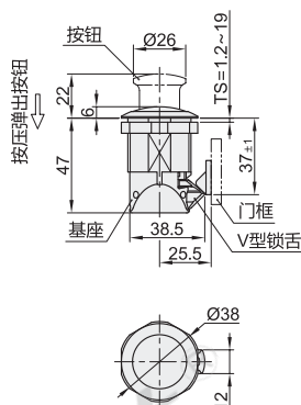
拉起按钮型 XBF05/06
