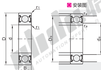
安装图
