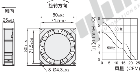
外形尺寸: 8025
