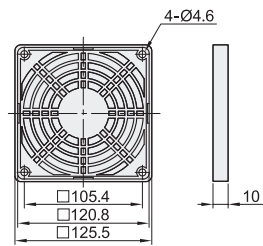
适用风扇外形尺寸: 120
