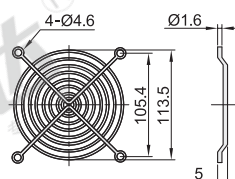
适用风扇外形尺寸: 120
