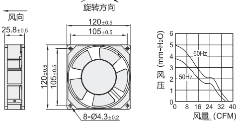
外形尺寸: 12025B
