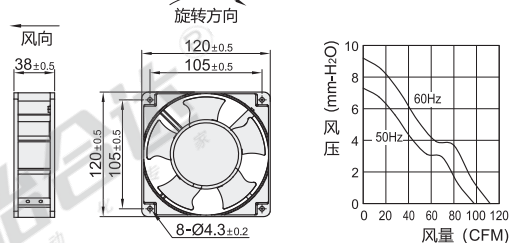
外形尺寸: 12038
