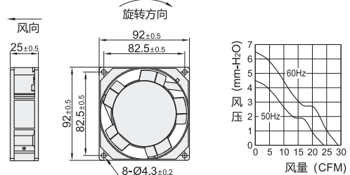
外形尺寸: 9225
