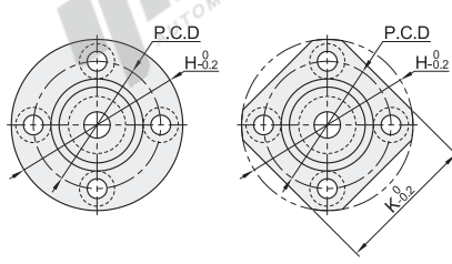
圆法兰 E-BFR01/02/03/04/06
