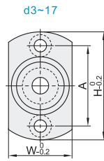
对边法兰 E-BFR21/22/23/24/26
