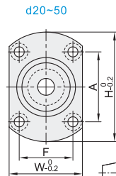
对边法兰 E-BFR21/22/23/24/26
