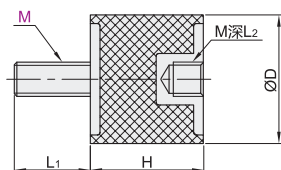
圆柱型 NHE02/08
