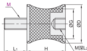
腰型 NHE12
