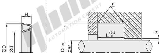
安装图例(开放式沟槽)
