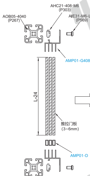
分解图
