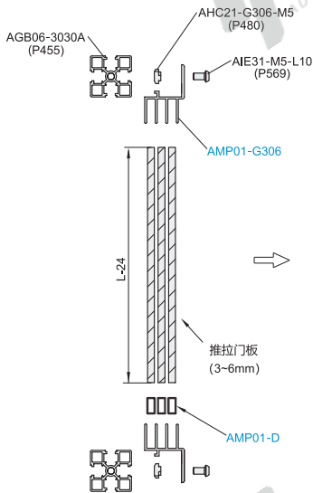
分解图
