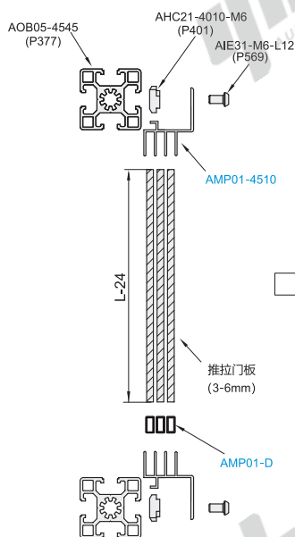
分解图
