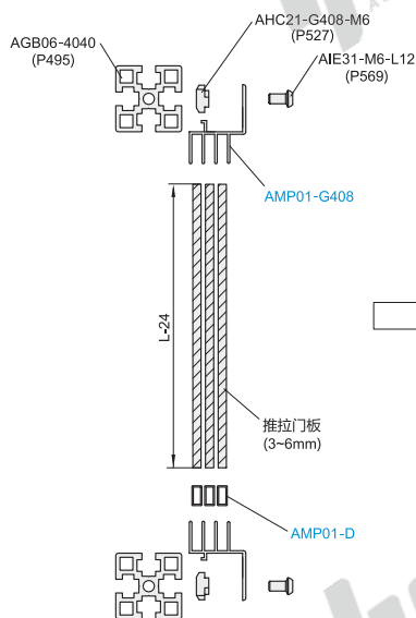
分解图
