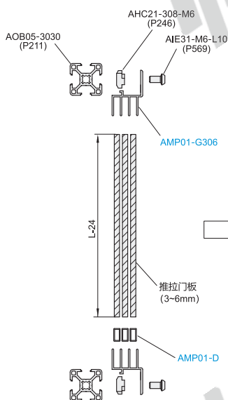
分解图
